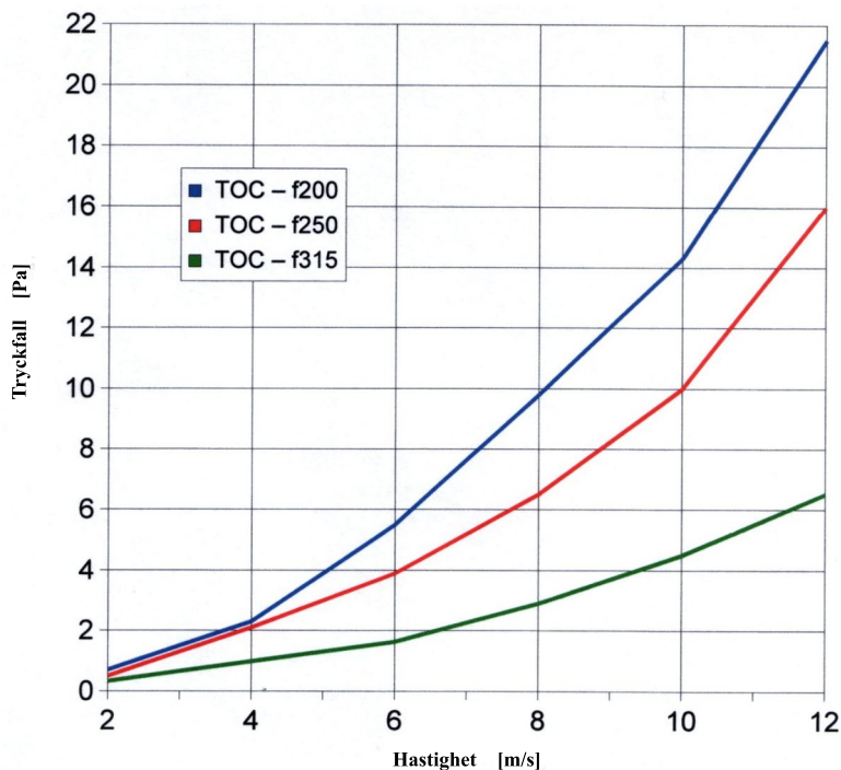
Figur 21. Exempel på hydrauliskt motstånd för ljuddämpare TOC (längd l = 900 mm).
